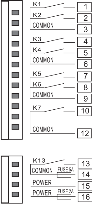
接線位置圖
