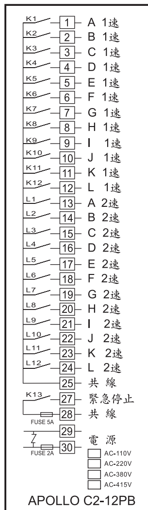
解碼繼電器板(REV:3.21)
