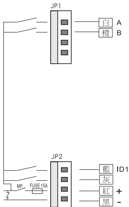
接線位置圖
