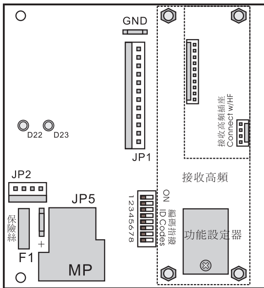
解碼驅動板
