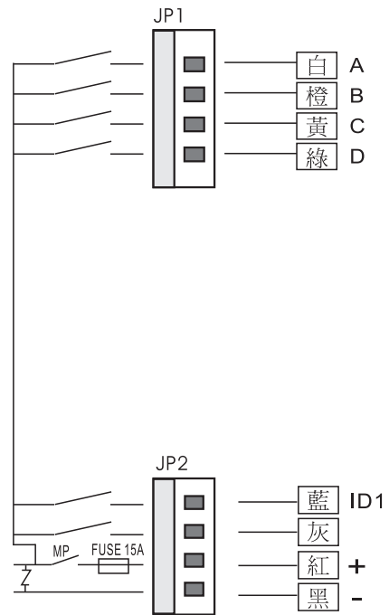
接線位置圖
