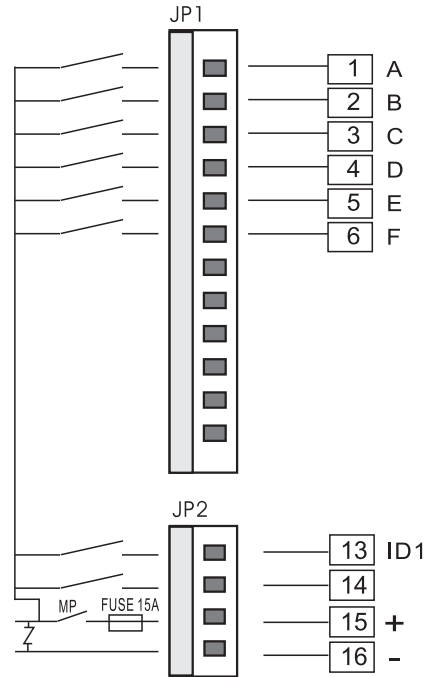
接線位置圖
