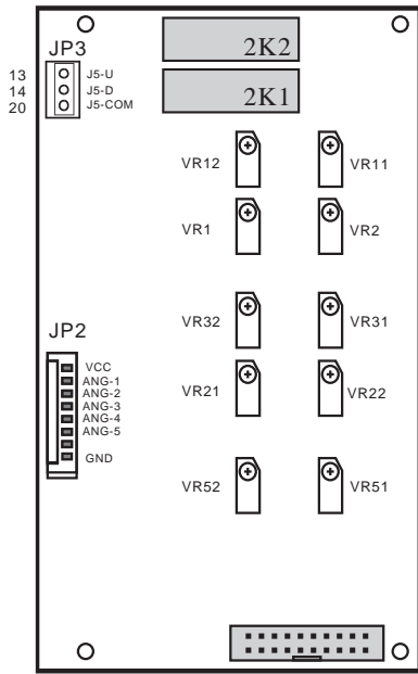
變頻用比例擴充繼電器板
