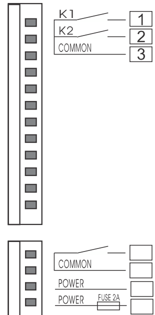
接線位置圖
